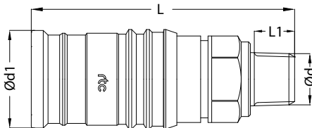
Socket / Kuplungen
