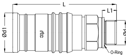
Socket / Kuplungen
