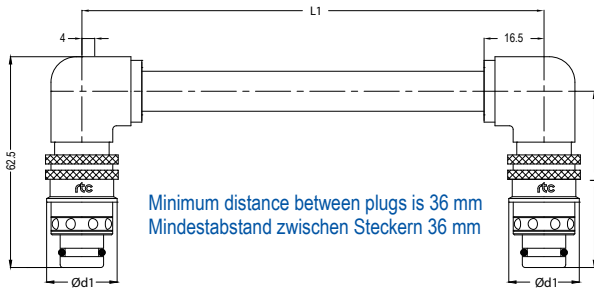
Plug / Stecker
