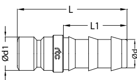
Plug / Nippel
