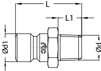
Plug / Nippel
