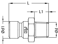
Plug / Nippel
