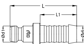
Plug / Nippel
