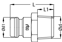
Plug / Nippel
