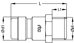
Plug / Nippel
