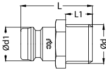
Plug / Nippel
