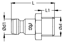
Plug / Nippel
