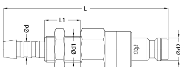
Plug / Nippel
