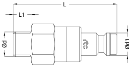
Plug / Nippel
